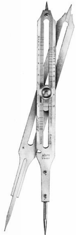
Reduktionszirkel 1092 Fr. 165.—
