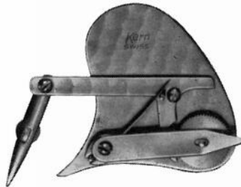
Doppelkurvenfeder 1053 Fr. 39.50
